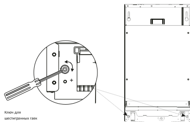
Ключ для шестигранных гаек CR-V 4 мм
