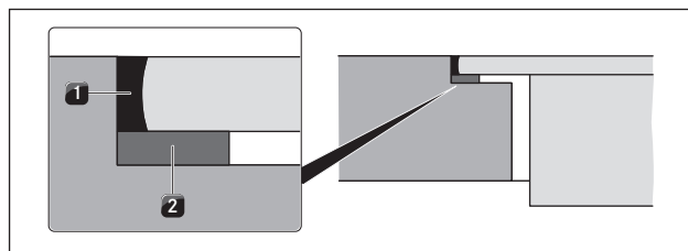
рис. 5.6 Уплотнительная лента при монтаже вровень с поверхностью
