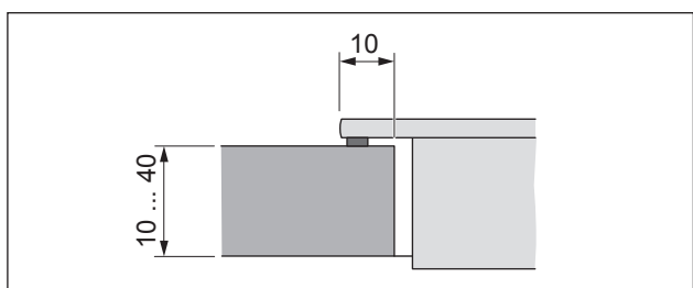
рис. 5.5 Вырез при навесном монтаже
