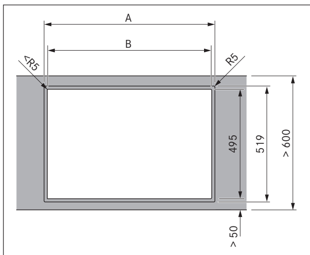
рис. 5.2 Монтаж вровень с поверхностью
