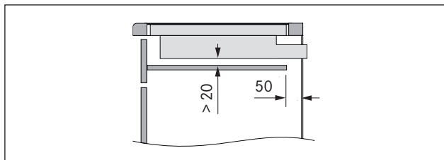
рис. 5.8 Защитная панель для кабеля и вентиляция: вид сбоку
