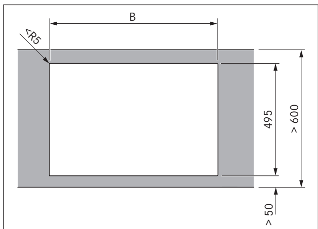
рис. 5.4 Навесной монтаж
