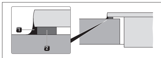
рис. 5.7 Уплотнительная лента при навесном монтаже
