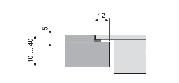
рис. 5.3 Размер паза в вырезе
