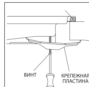
УПЛОТНИТЕЛЬ
