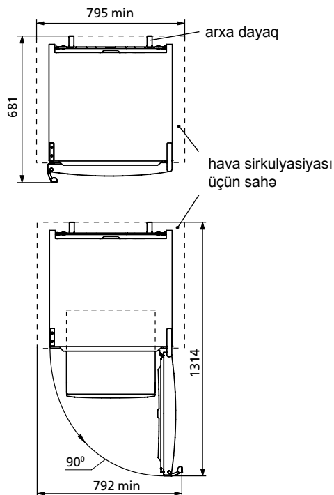
Rəsim 2 — Soyuducu (üstdən görünüşü) bölümünün qapısı
