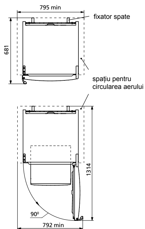
Imagine 2 — Frigider (vedere de sus)
