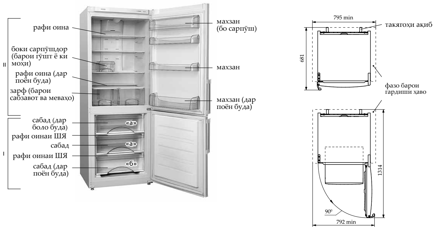
Расми 2 – Яхдон (намуди он аз боло)
