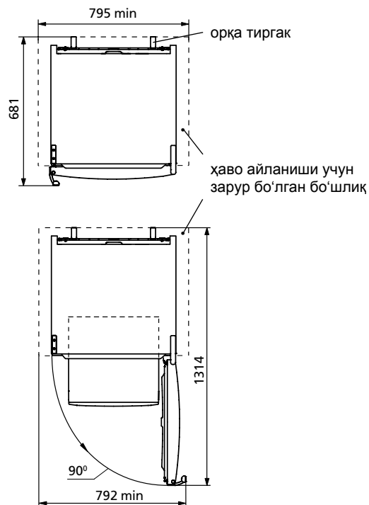
2-расм — Совутқич (уст қисмидан кўриниши)
