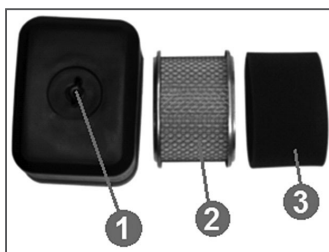
Рис. 21 Конструкция воздушного фильтра
