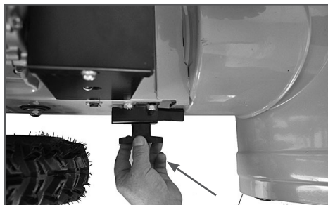
Рис. 10 Закрепление снегоотбрасывателя
