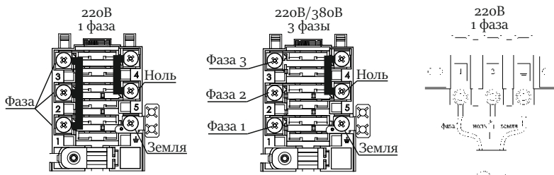
Рисунок 6 - Подключение кабеля электроплиты к электросети
