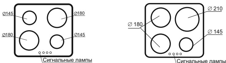
Рисунок 4 - Конфорочная панель. Зоны нагрева конфорок
