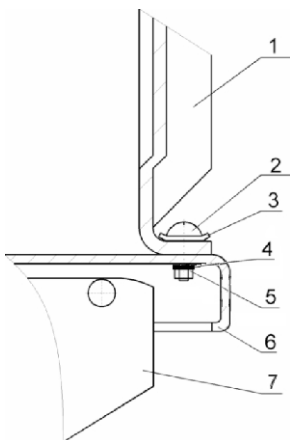
Рисунок 7 - Установка щитка на плиту
