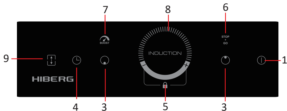
для модели HIBERG i-MS 3029 B
