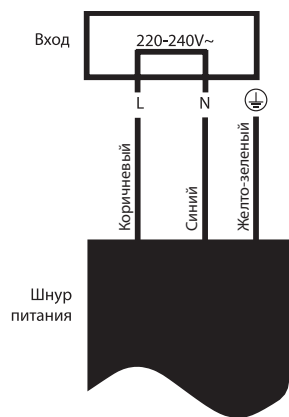
для моделей HIBERG i-MS 3029 B / Y
