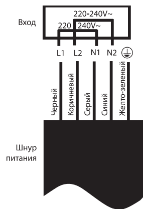
для моделей HIBERG i-MS 6049 B / Y
