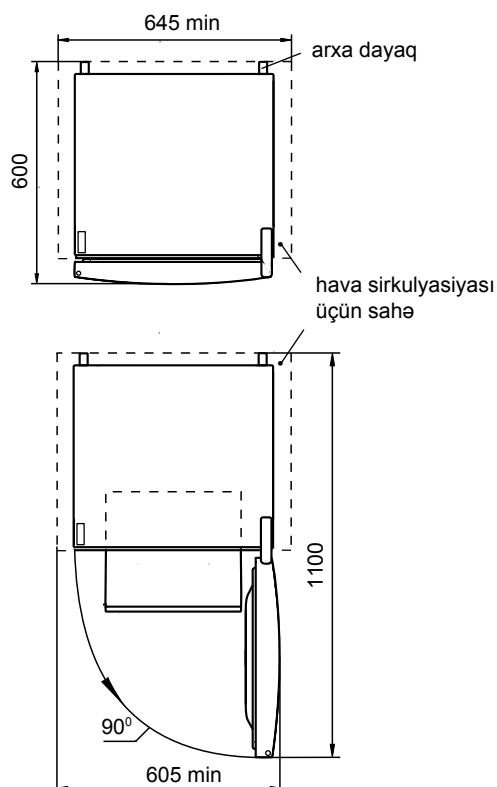
Şəkil 2 – Soyuducu (yuxarıdan görünüş)
