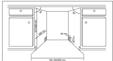
Габариты моделей
