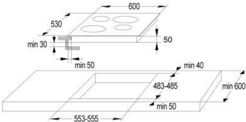
Рис. 1. Подготовка столешницы к монтажу.
