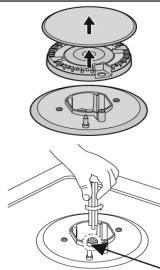
Инжектор
