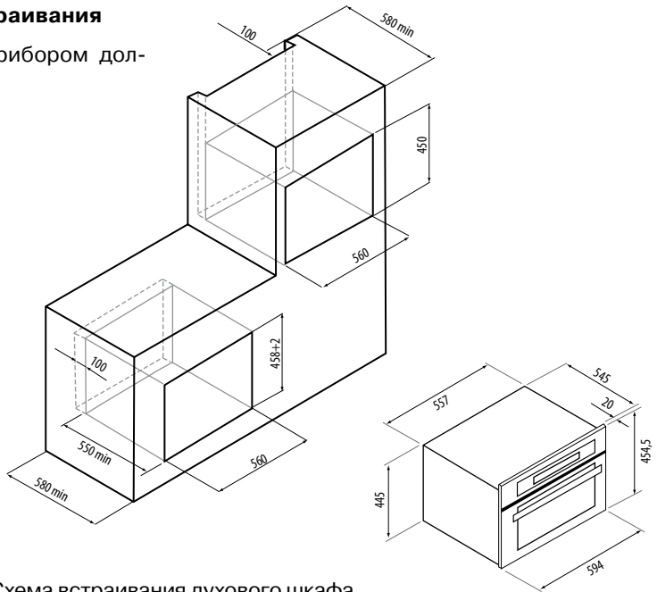
Схема встраивания духового шкафа.
