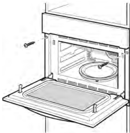
Крепление духового шкафа к мебели.
