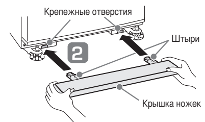
Крепежные отверстия
